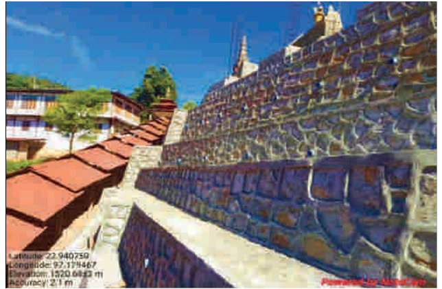
နမ့်ဆန်မြို့နယ်၊ ဘုရားကြီးကျေးရွာ ဘုန်းကြီးကျောင်း စေတီရင်ပြင်ဘေးတွင် မြေထိန်းနံရံ ၇၅ ပေ x ၂၀ ပေ တည်ဆောက်ခြင်း
